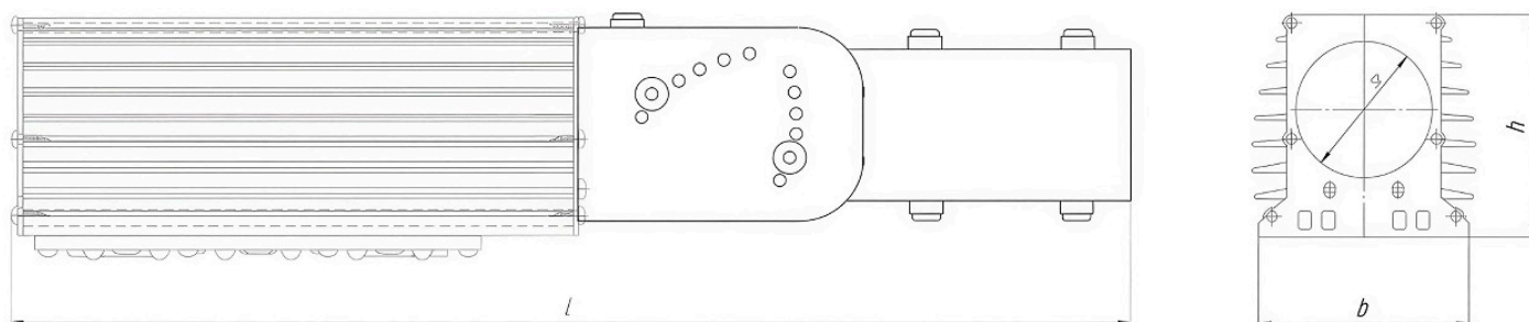
Рисунок 1 - Конструкция светильника
