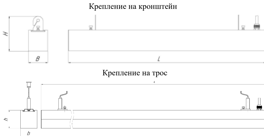
Рисунок 1 – Конструкция светильника
