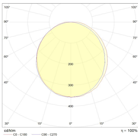
Рисунок 1 - КСС светильника в двух меридиональных плоскостях: 0-180 и 90-270.
