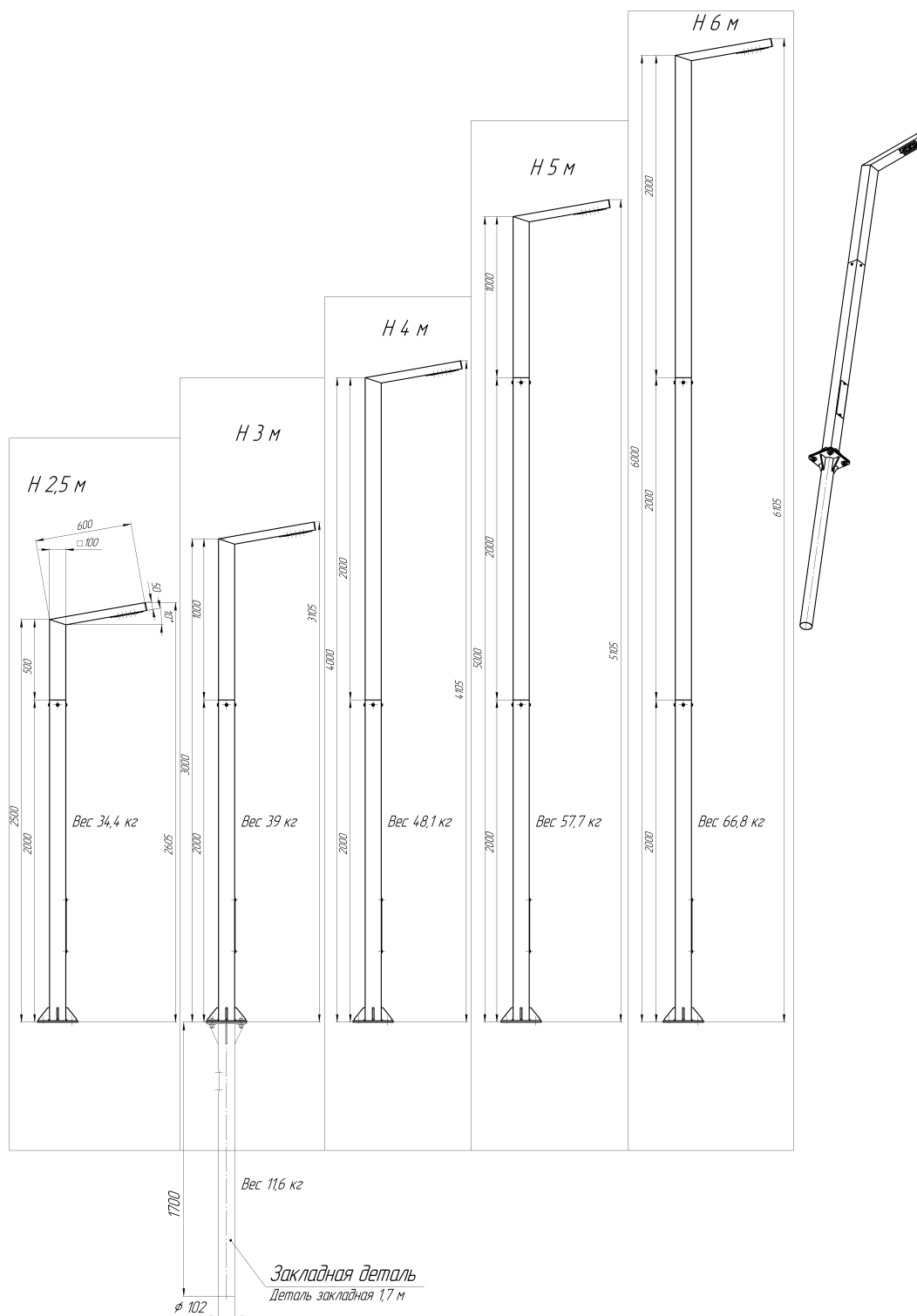
Рисунок 1 - Конструкция светильника
