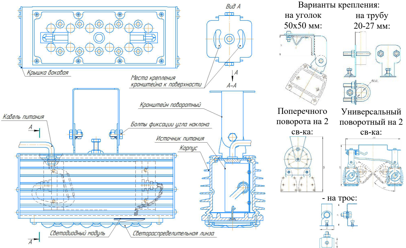
Рисунок 1 – Конструкция светильника
