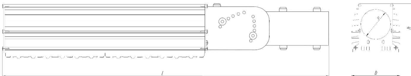
Рисунок 1 - Конструкция светильника
